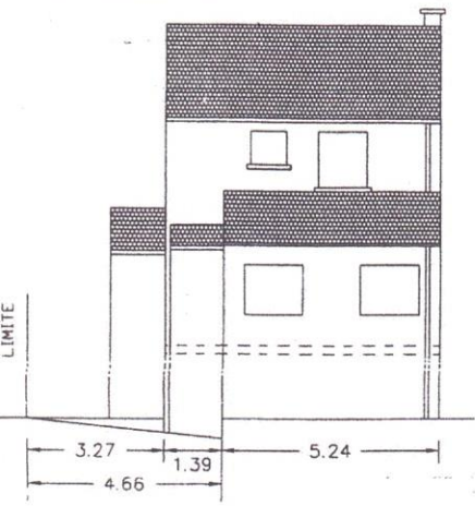
FACADE ARRIERE APRES TRAVAUX ECH : 1/100
