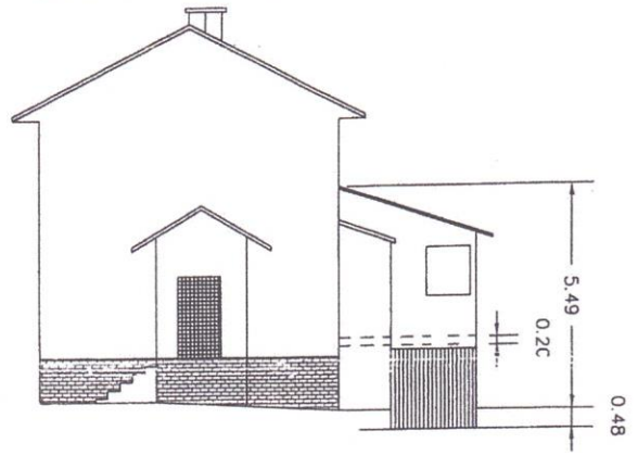
PIGNON APRES TRAVAUX ECH : 1/100
