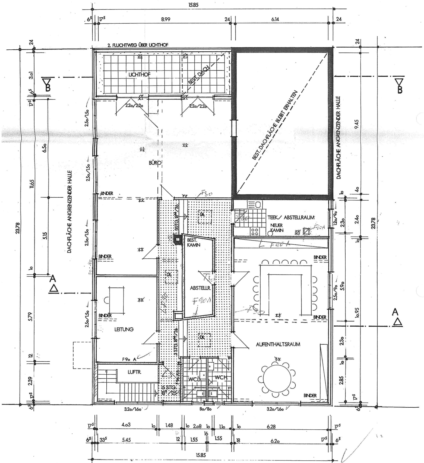
GRUNDRISS OBERGESCHOSZ M 1:100
