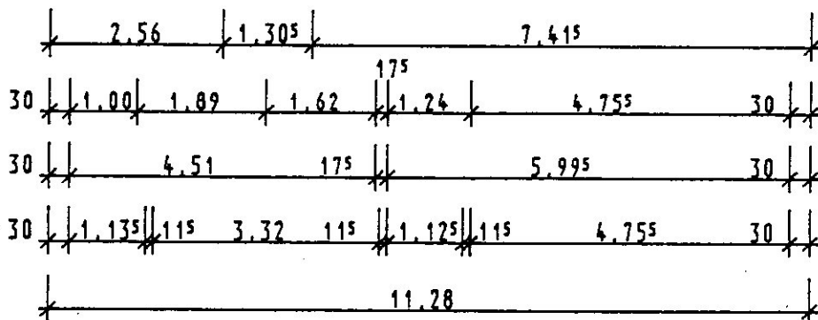
GRUNDRISS DACHGESCHOSS
