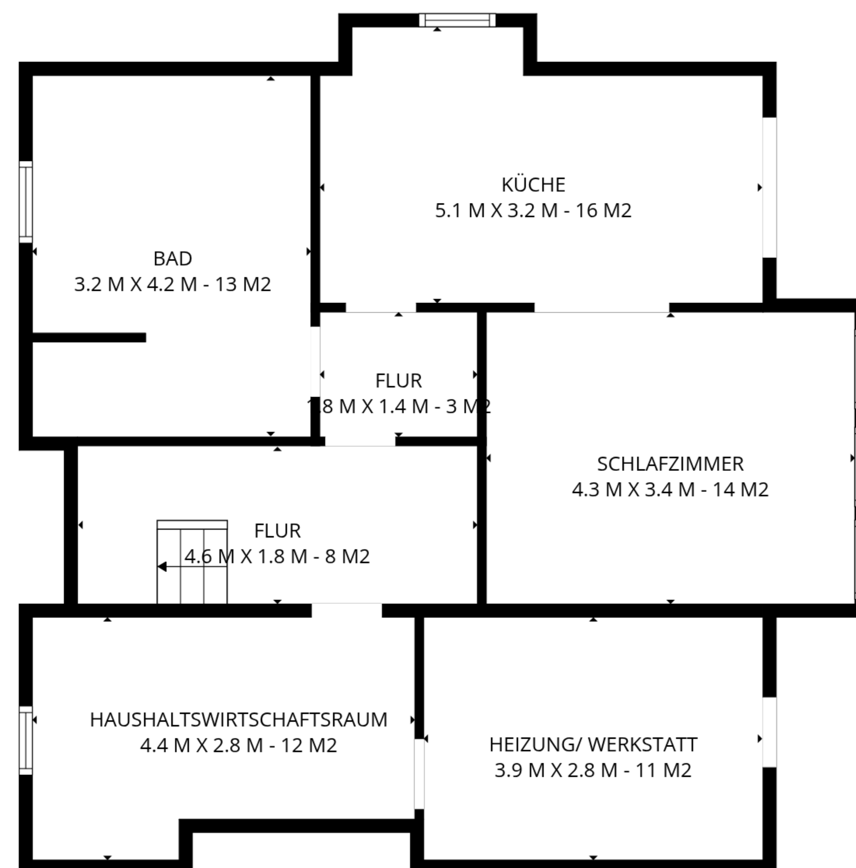
ERDGESCHOSS
