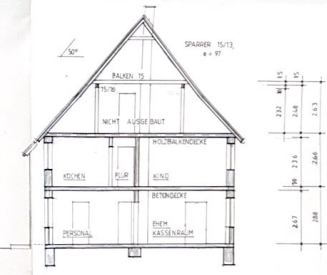
SCHNITT 1-1 1:100
