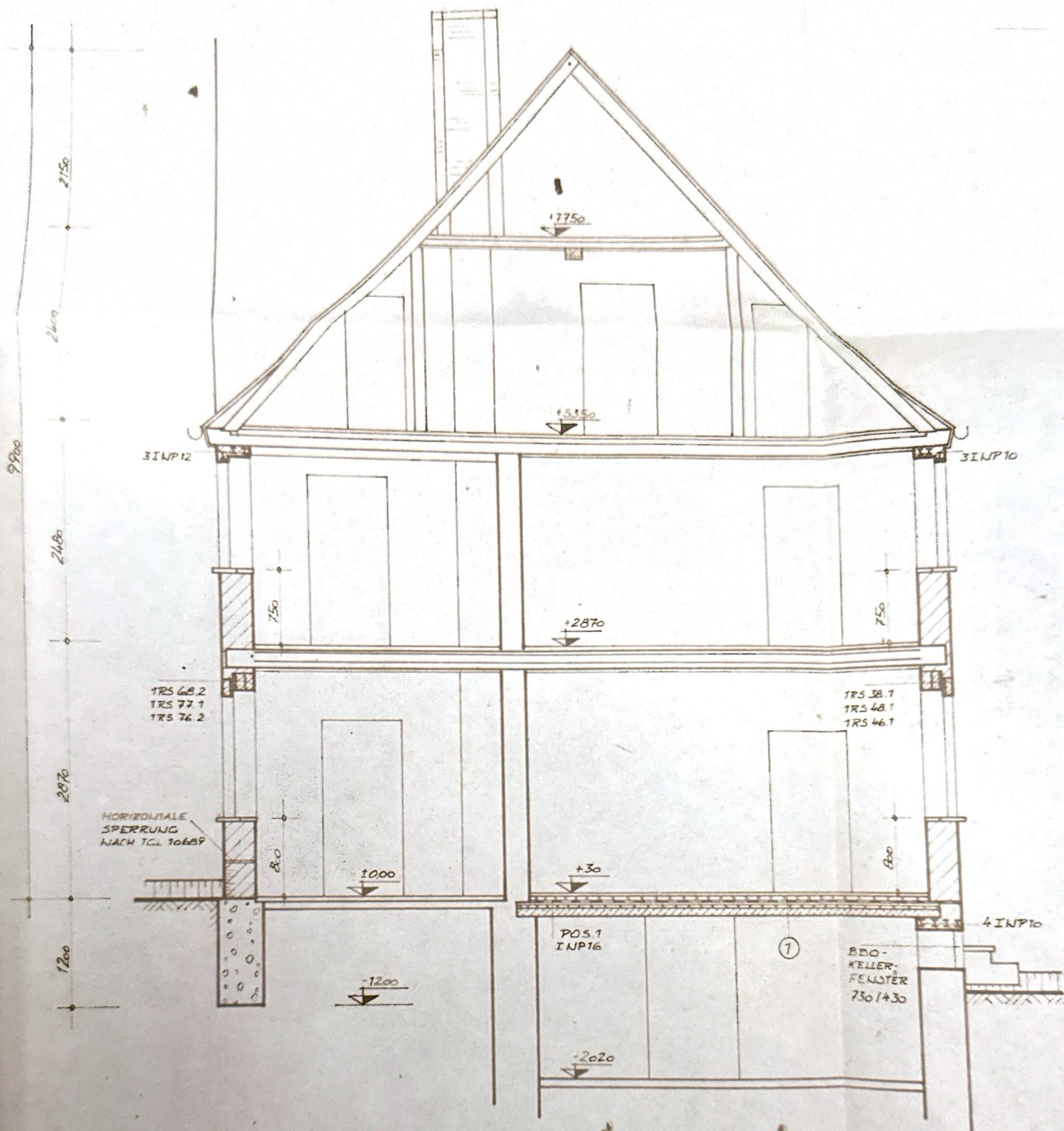
SCHNITT A-A - NEU-
