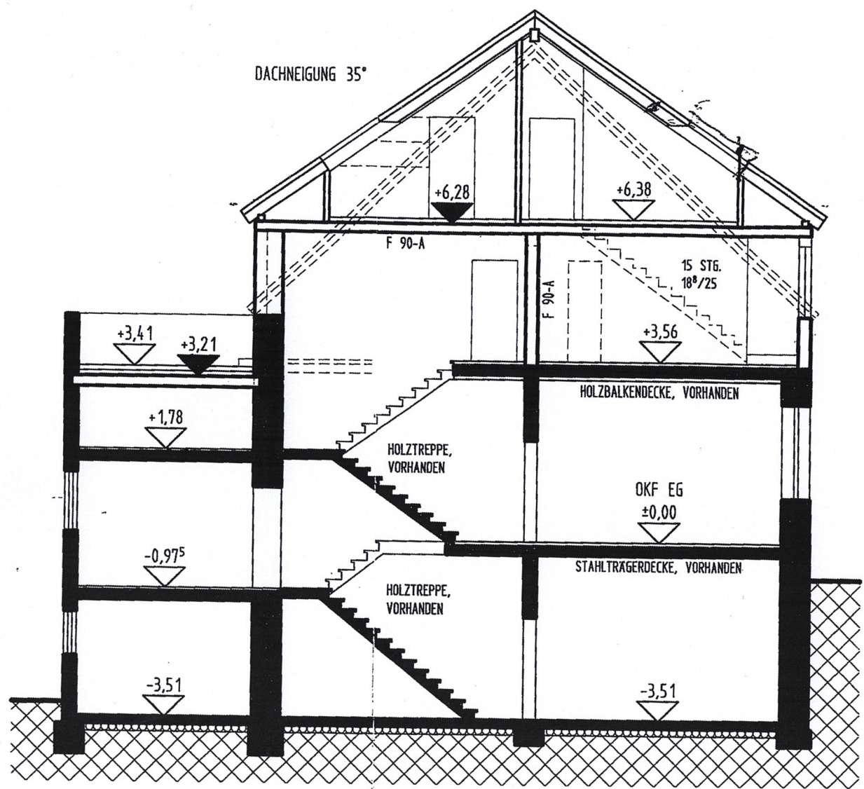
ССЧНИТТ А-А М 1:100
