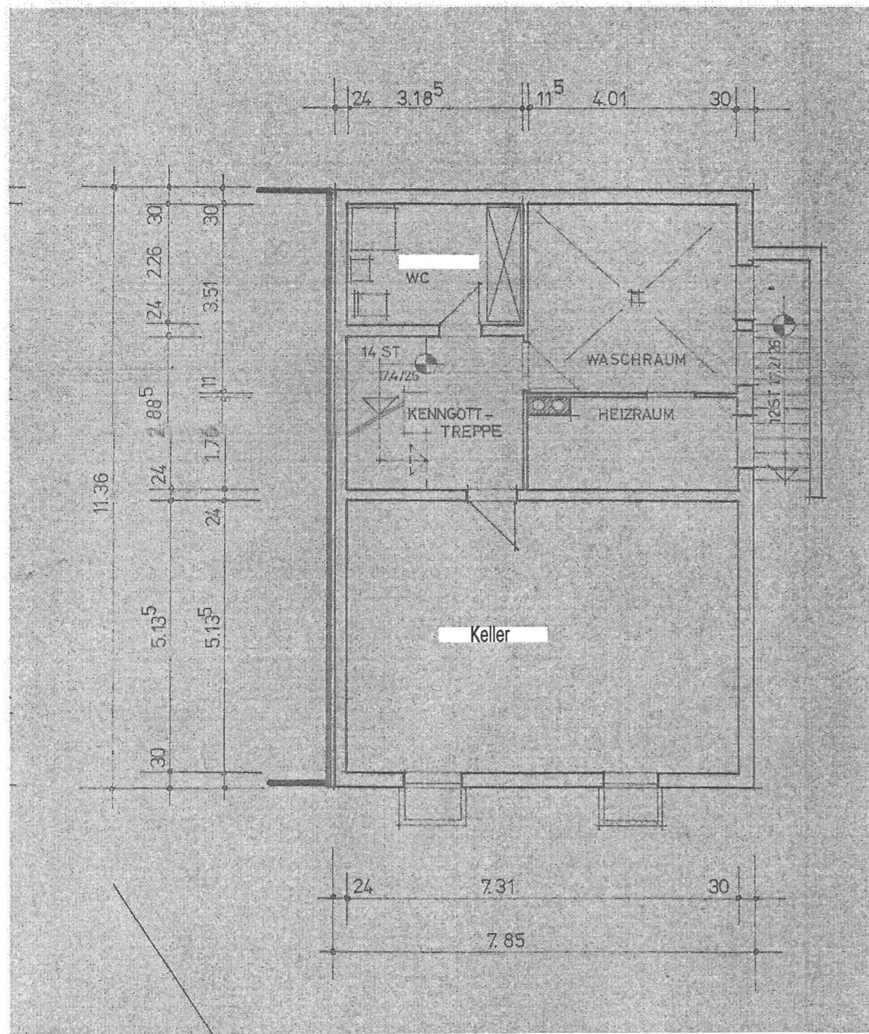
Grundriss Kellergeschoss
