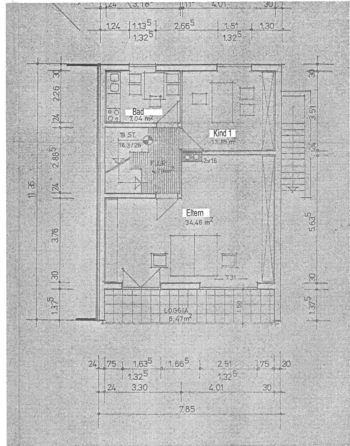
Grundriss Obergeschoss
