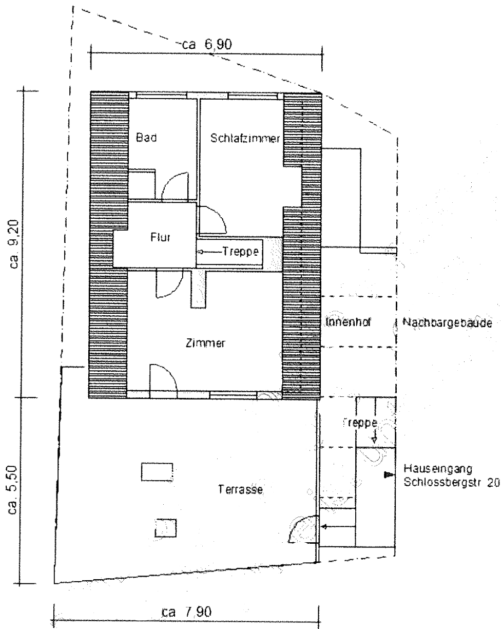
Grundriss-Schemaskizze des Sachverständigen; Dachgeschoss (ohne Maßstab)
