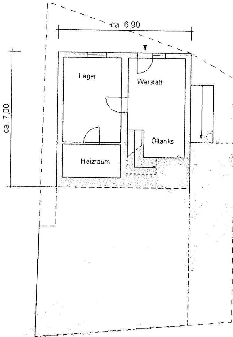
Grundriss-Schemaskizze des Sachverständigen; Untergeschoss/Keller (ohne Maßstab)
