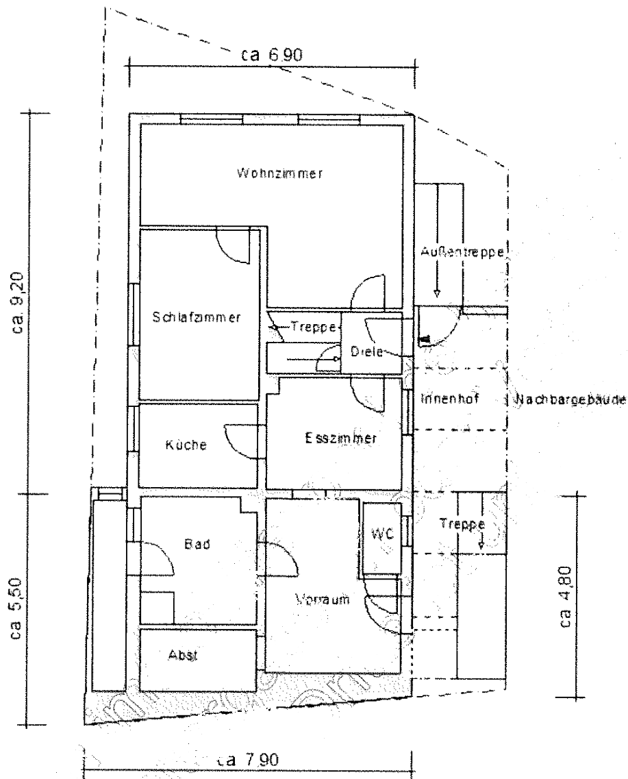
Grundriss-Schemaskizze des Sachverständigen; Erdgeschoss (ohne Maßstab)
