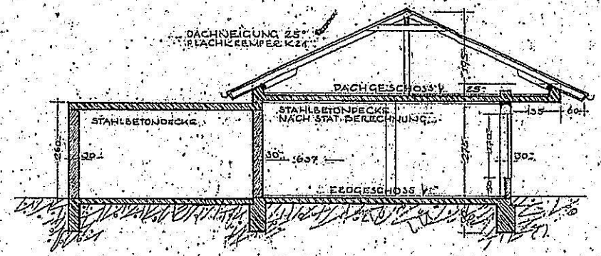
QUERSCHNITT C-D
