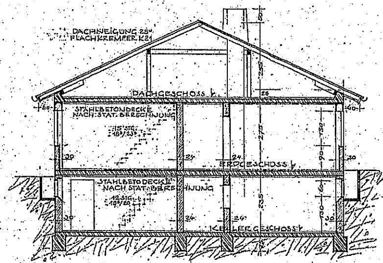
QUERSCHNITT A-B
