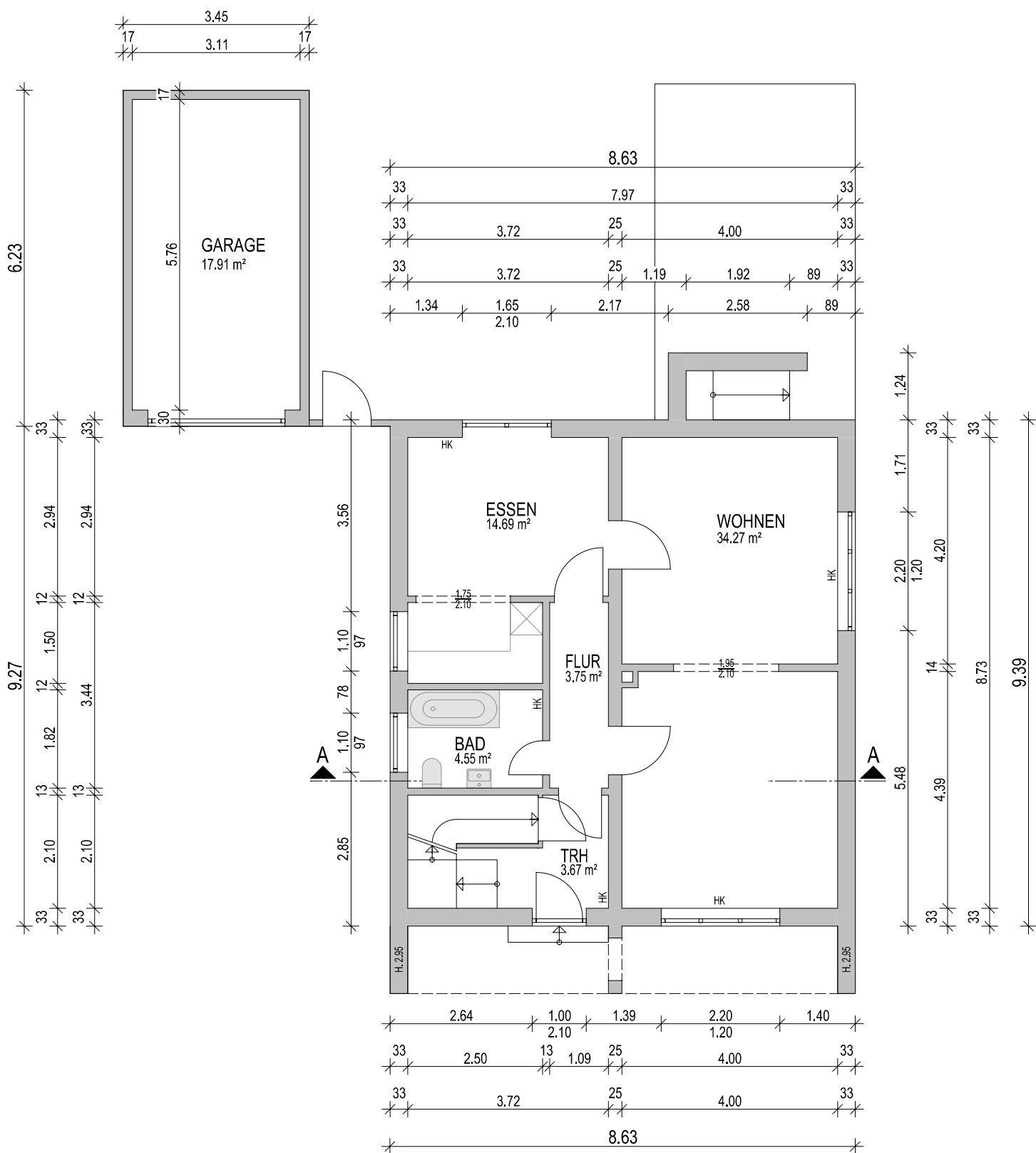
GRUNDRISS ERDGESCHOSS
