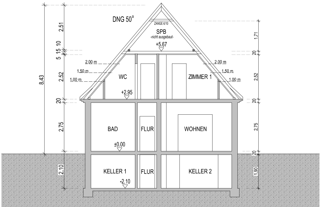
SCHNITT A-A
