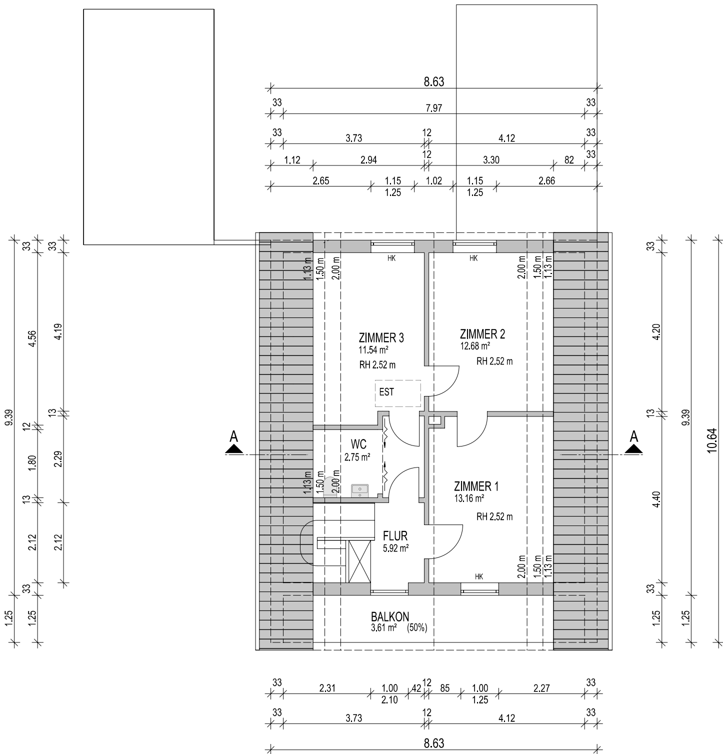
GRUNDRISS DACHGESCHOSS
