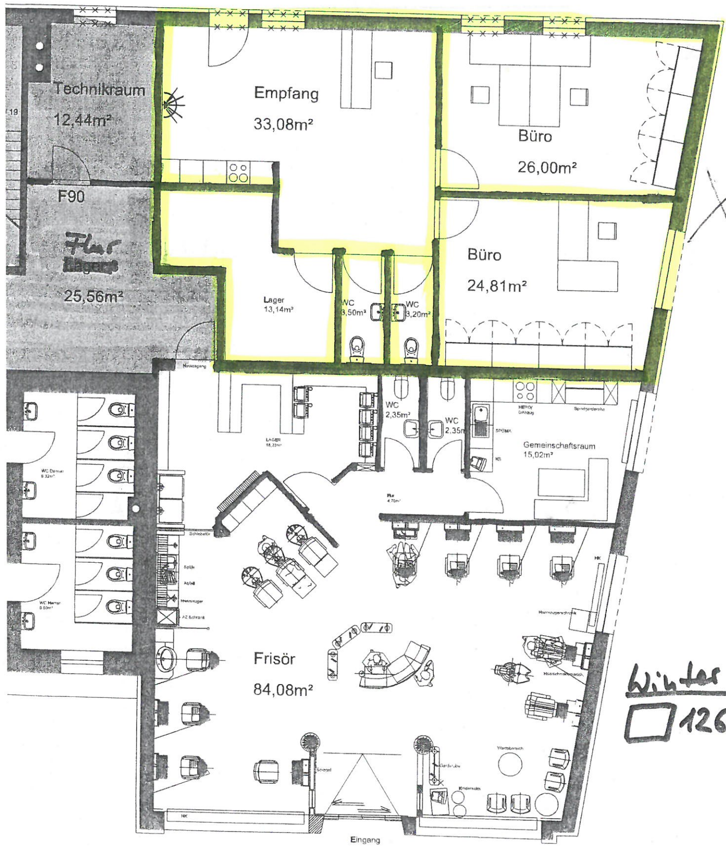
EG M1:100
