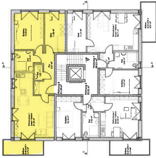
1.Obergeschoss
