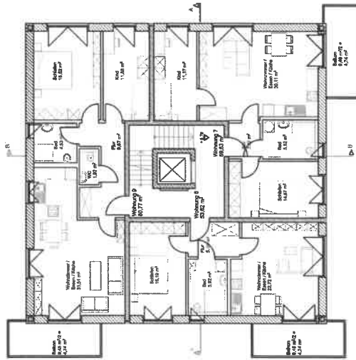
2.Obergeschoss
