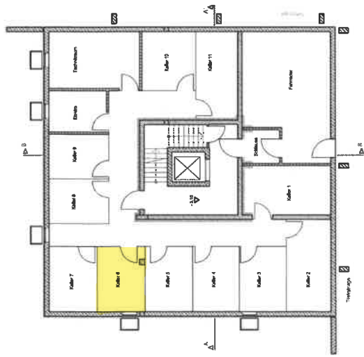
Kellergeschoss
