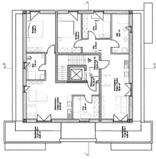
Dachgeschoss
