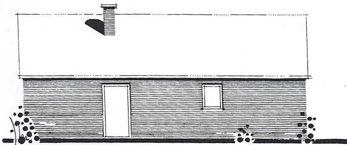
RÜCK-ANSICHT
