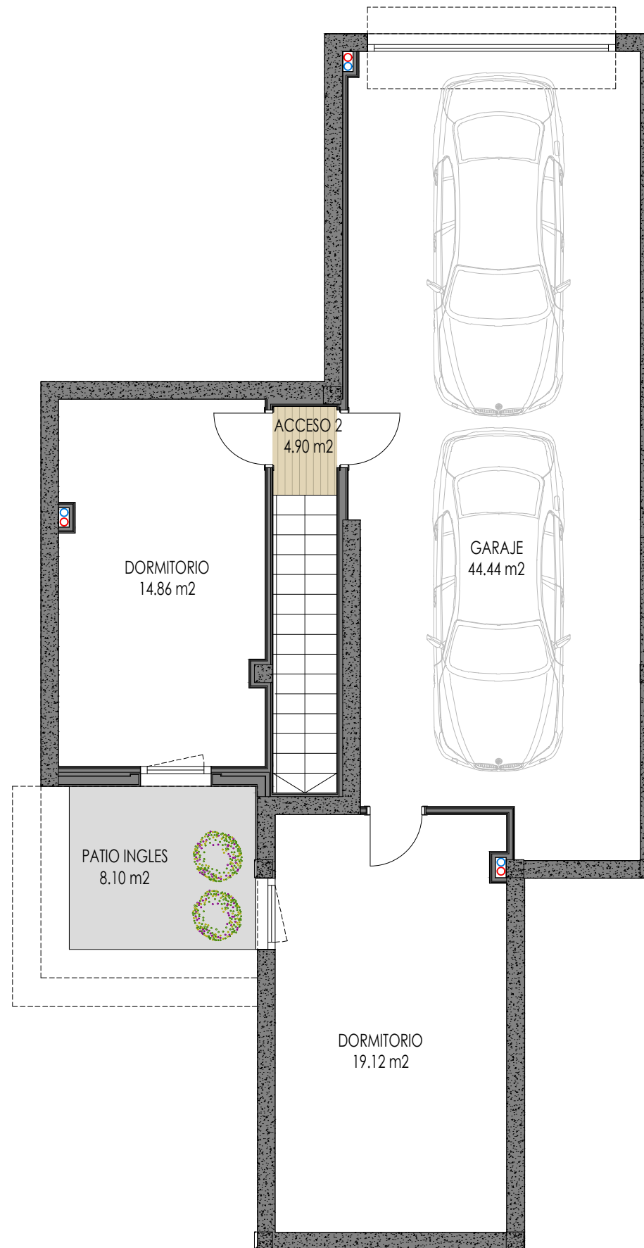
PLANTA SÓTANO
