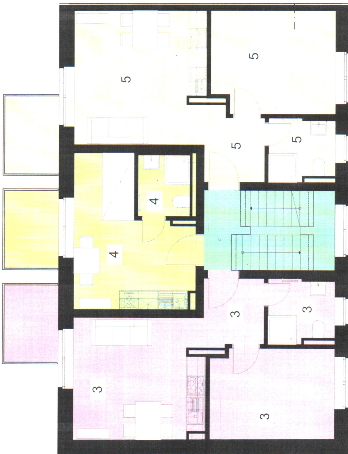
Grundriss 1.OG
