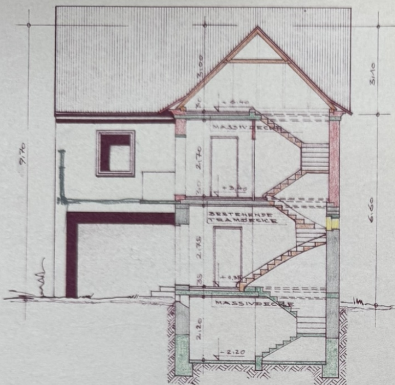
SNITT A-B
