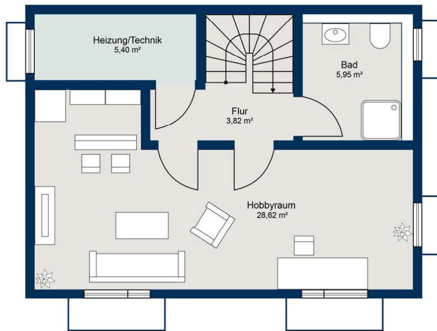
Untergeschoss
