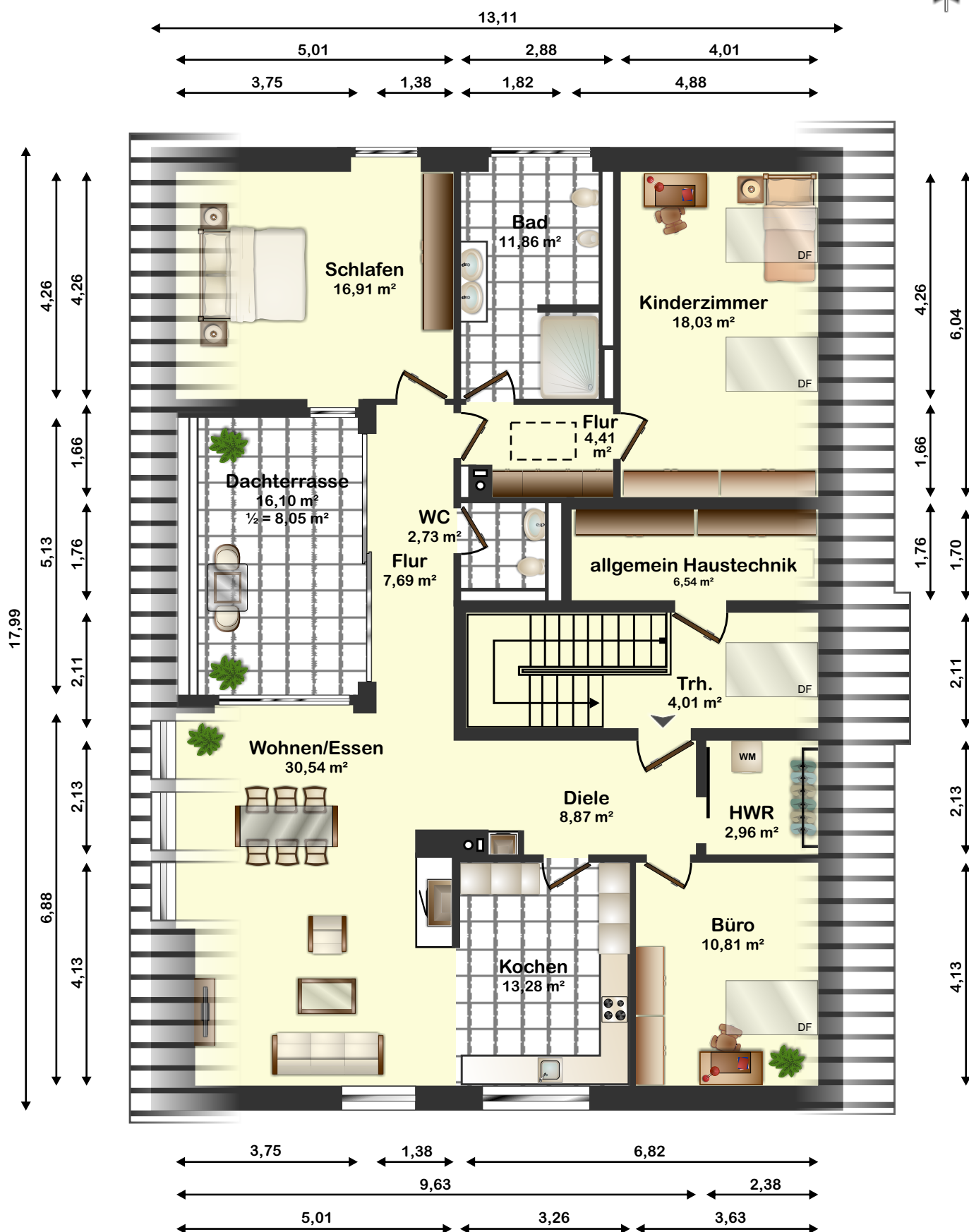
Dachgeschoss
