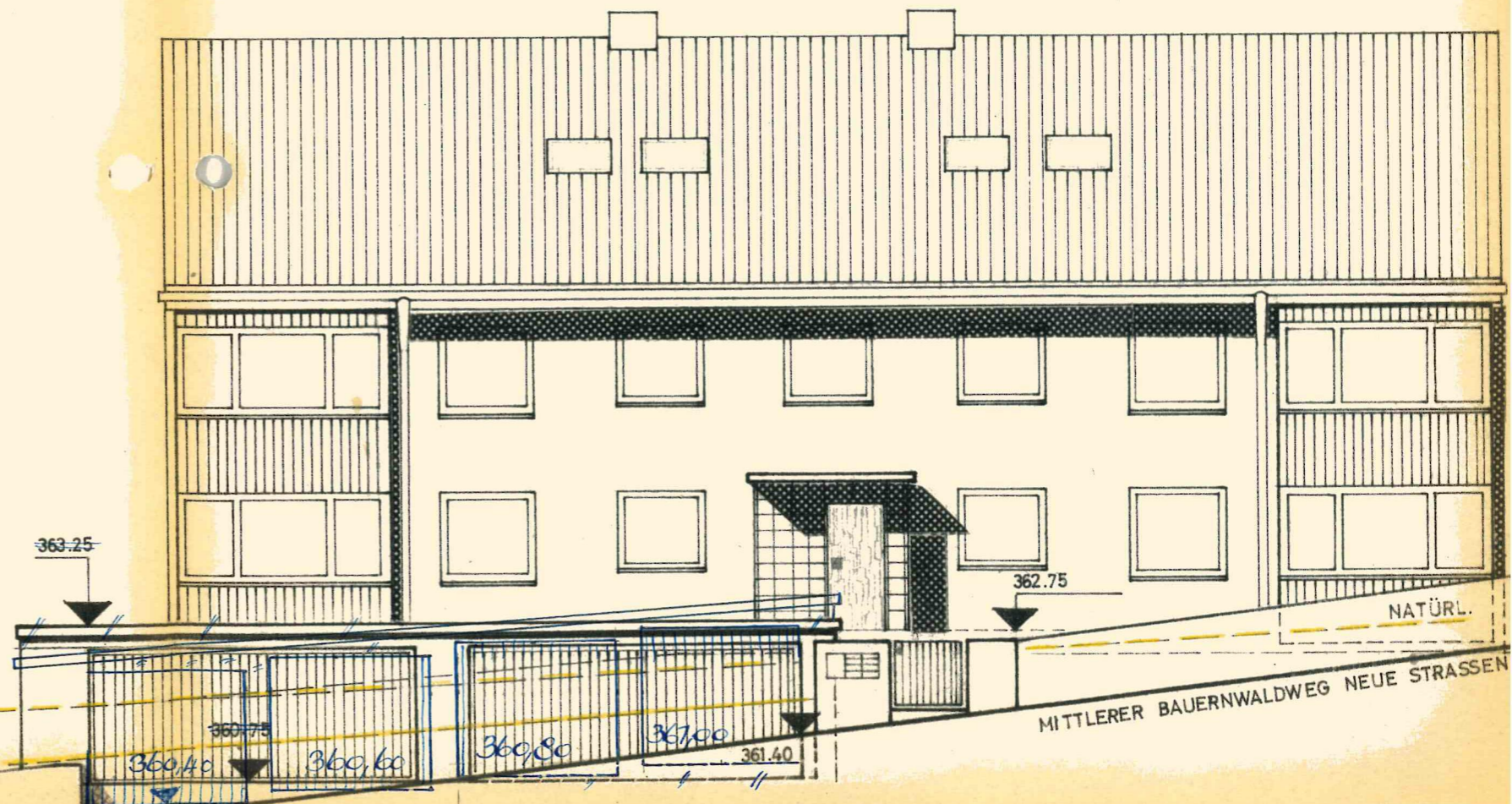
NORDANSICHT
