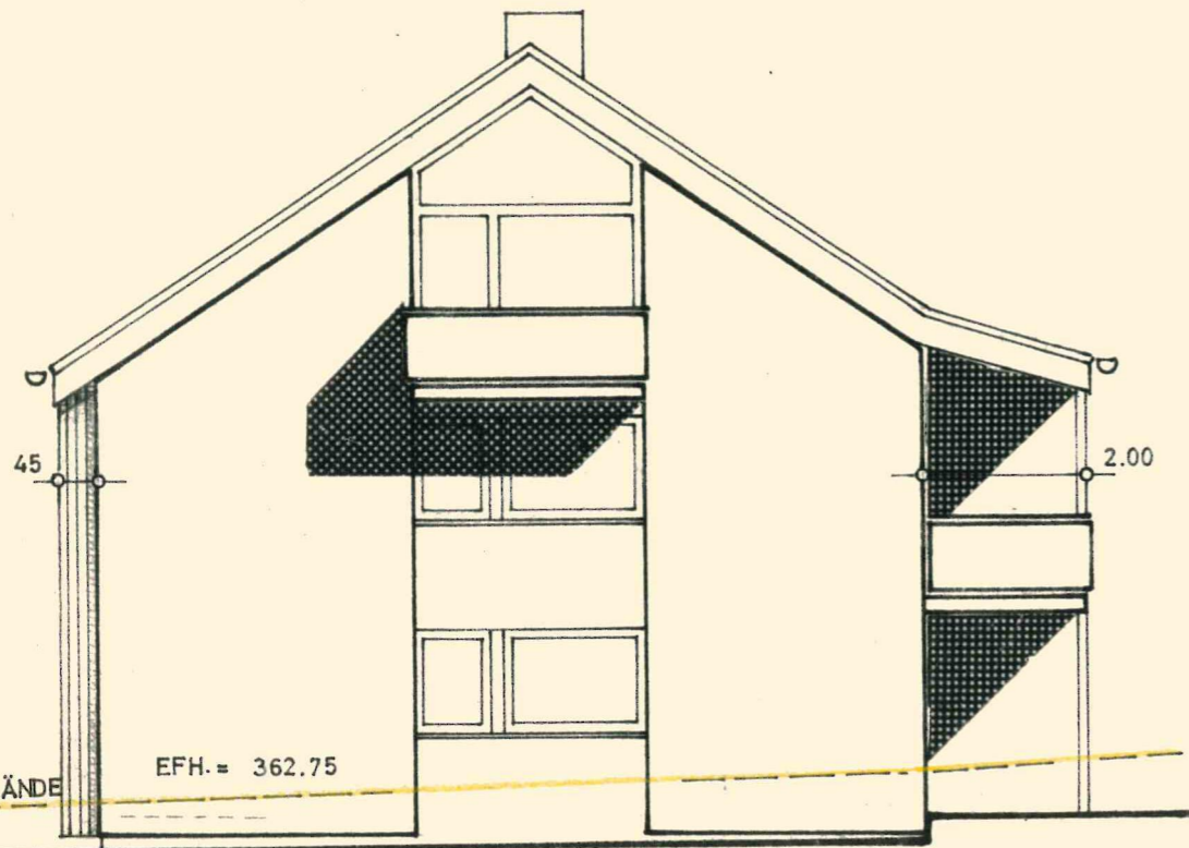
WESTANSICHT
