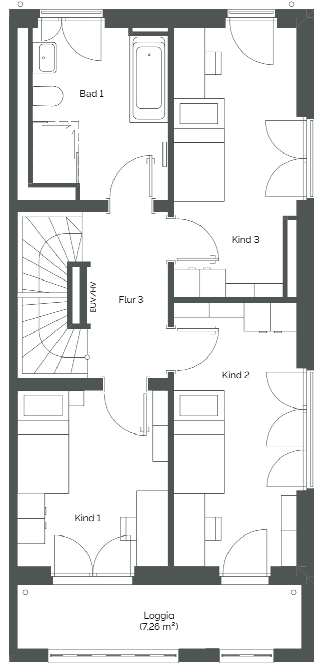
1. Obergeschoss
