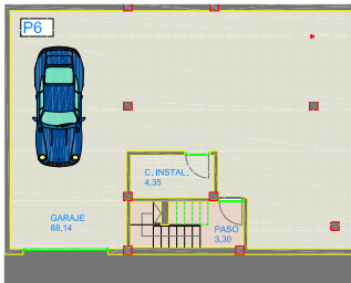
PLANTA SÓTANO GARAJE FLOOR
