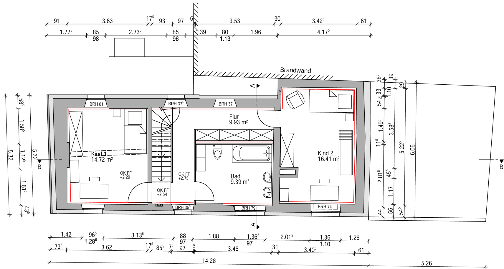
Obergeschoss Neuplanung
