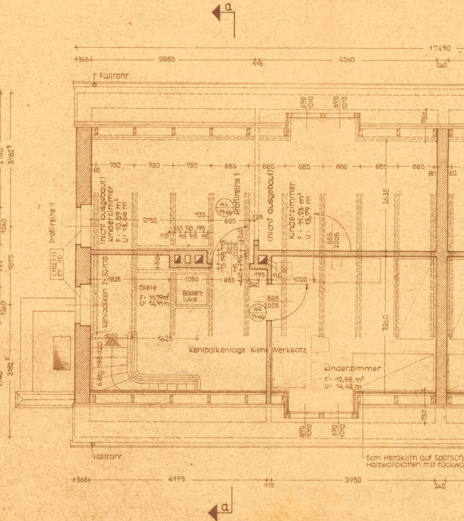
DACHGESCHOSS - GRUNDRISS
