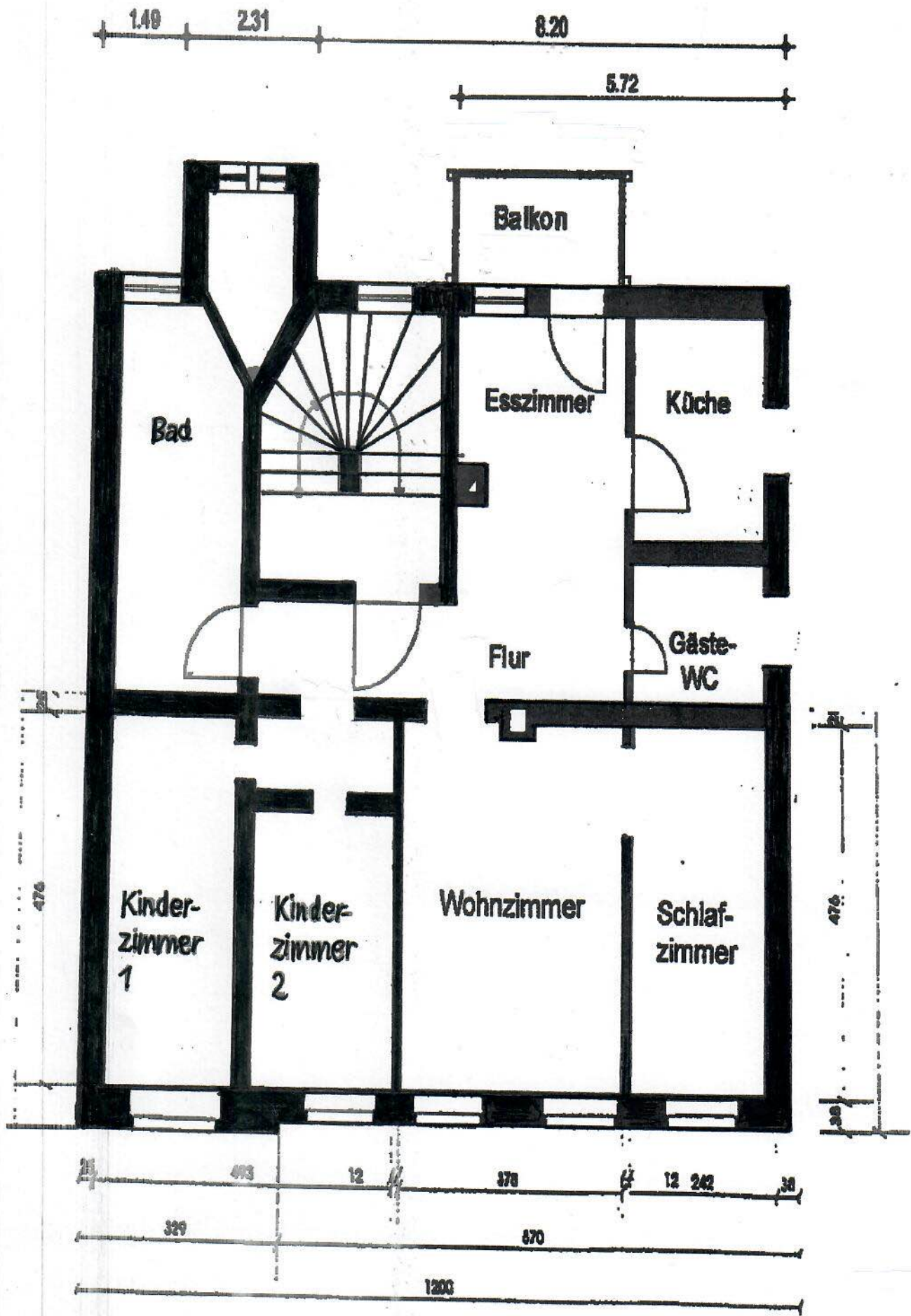
2. Obergeschoss
