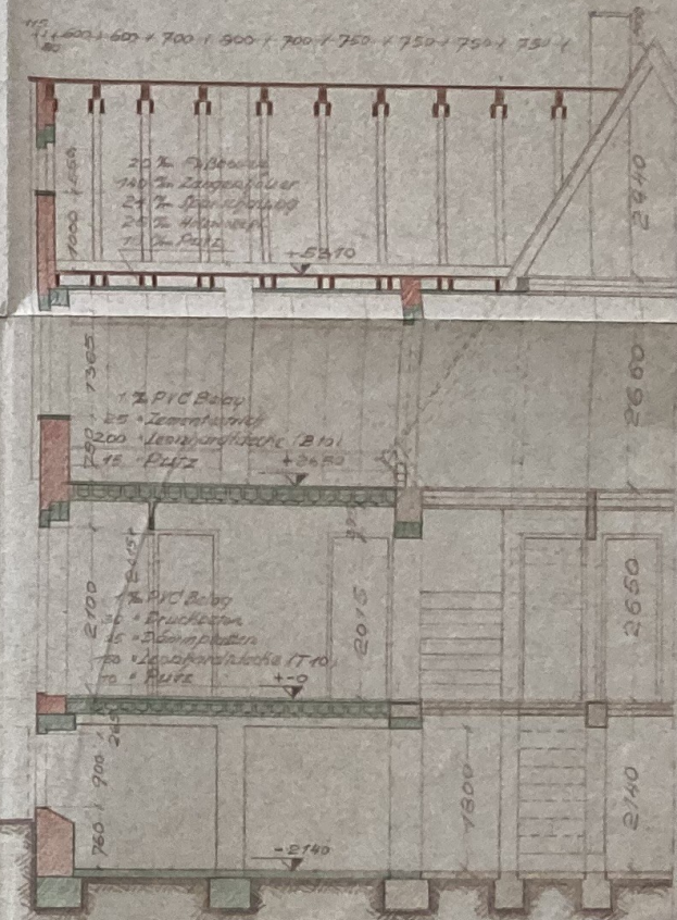
Schnitt C-D
