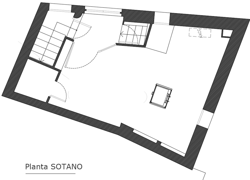
Planta BAJA
