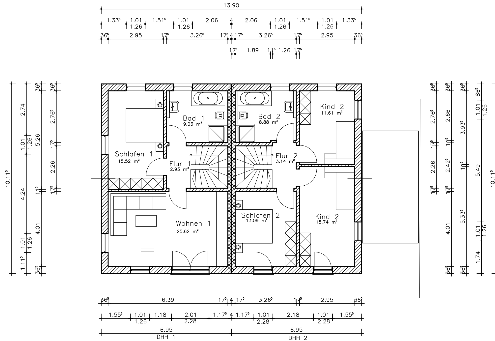
Obergeschoss – Grundriss
