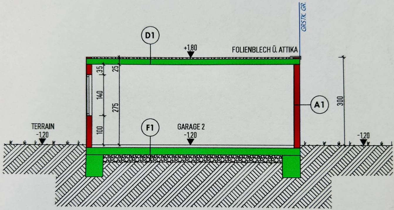
SCHNITT B-B
