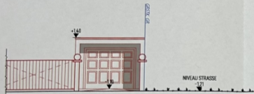
ANSICHT NORD
