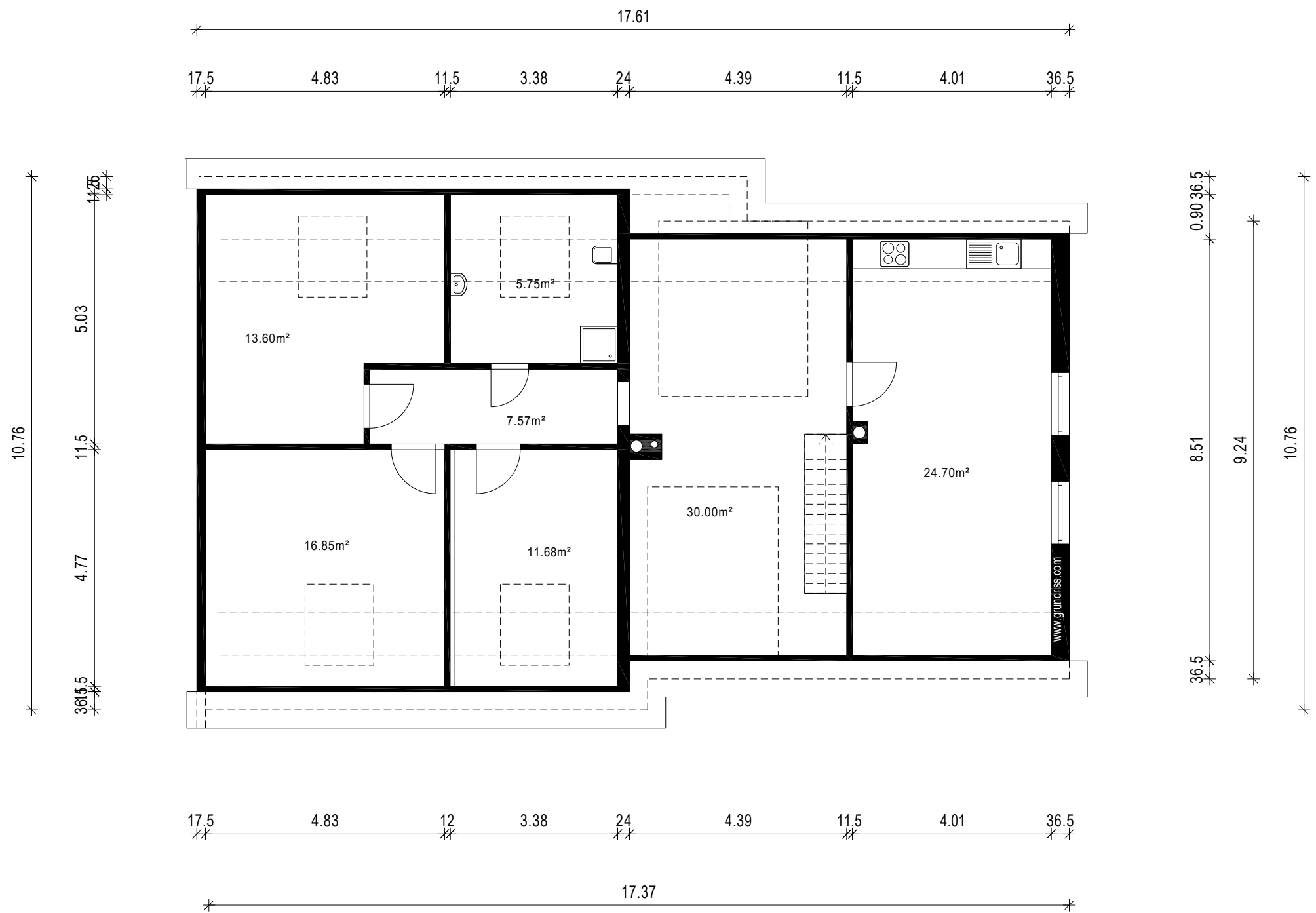
Dachgeschoss
