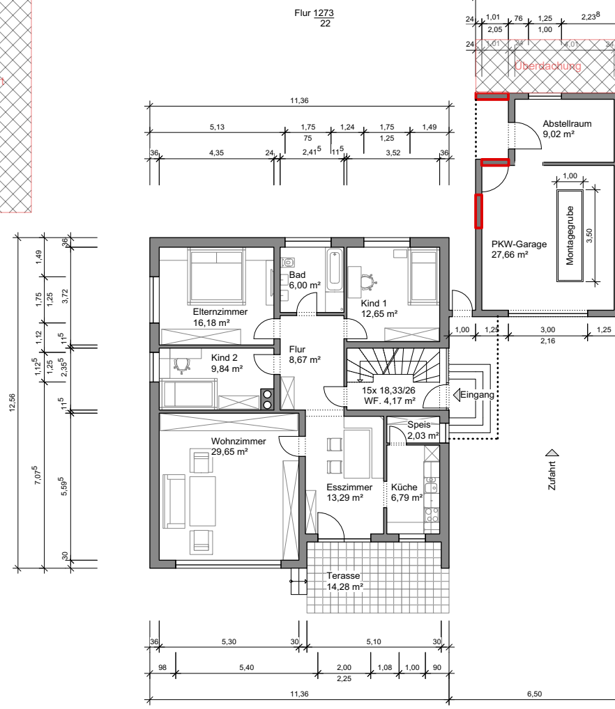
Grundriss Erdgeschoss
