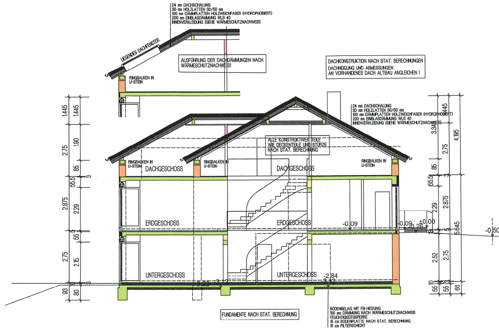
QUERSCHNITT 1-1
