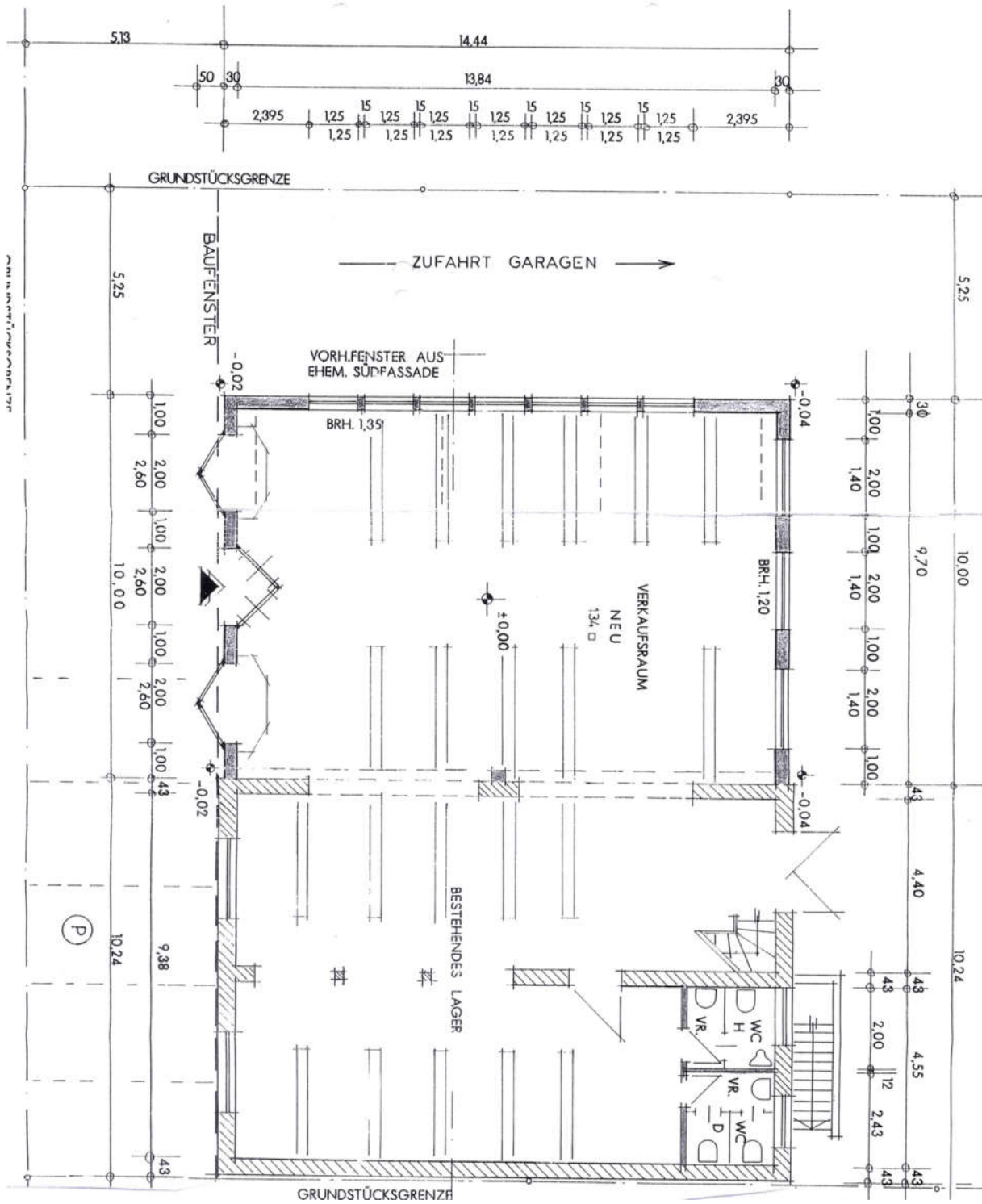
Grundriss Gewerbe (EG) vor Umbau!
