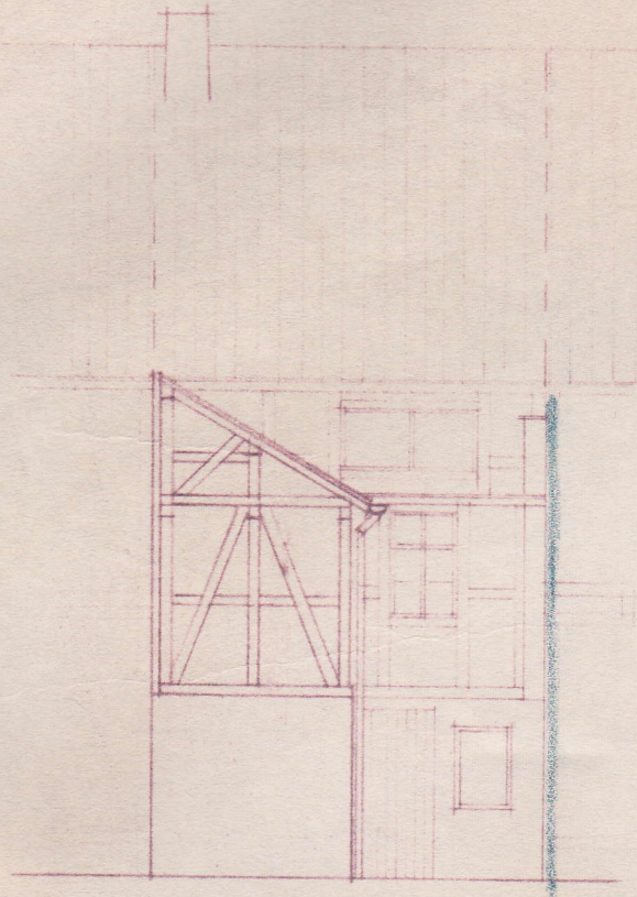
HOFANSICHT, ALT
