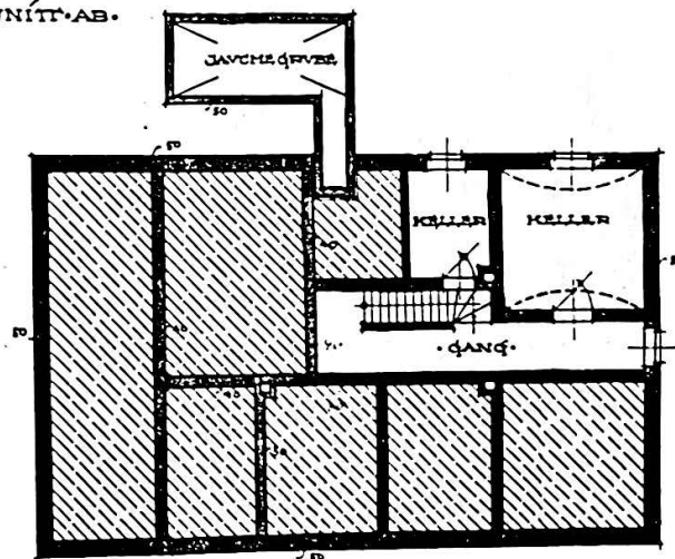
• KELLERGESCHOSS •
