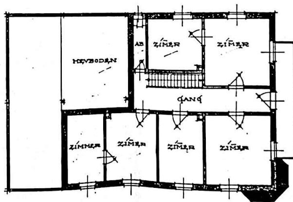
• OBERGESCHOSS •
