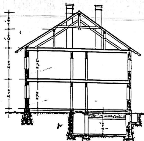
• SCHNITT-AB. •
