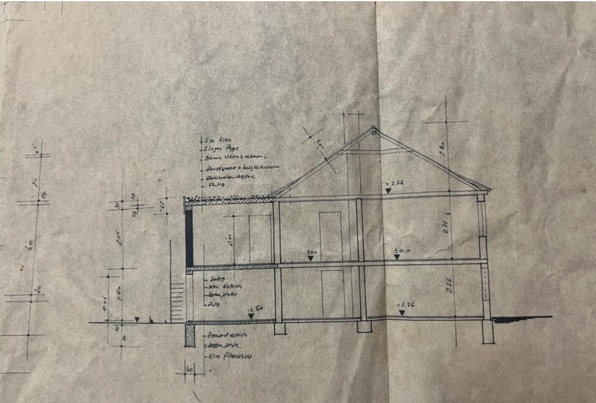
Querschnitt 1-1
