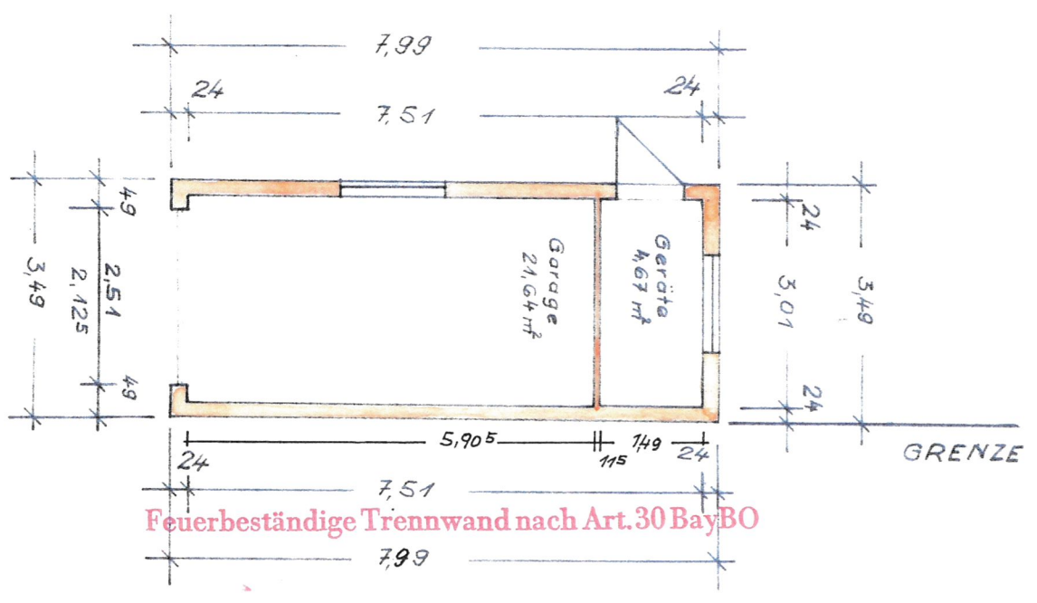
GRUNDRISS
