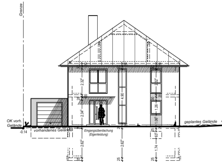
Westansicht
