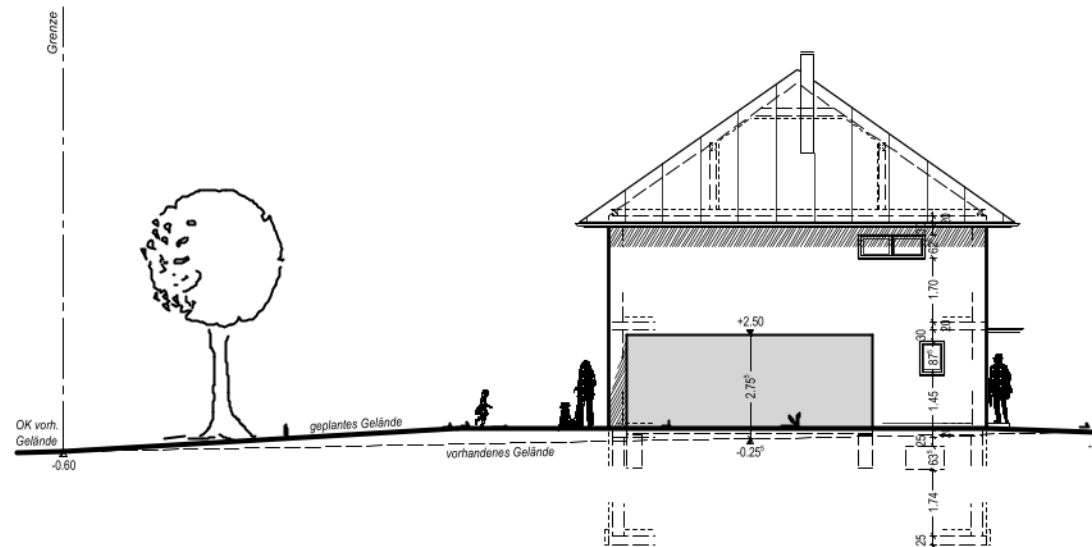
Nordansicht
