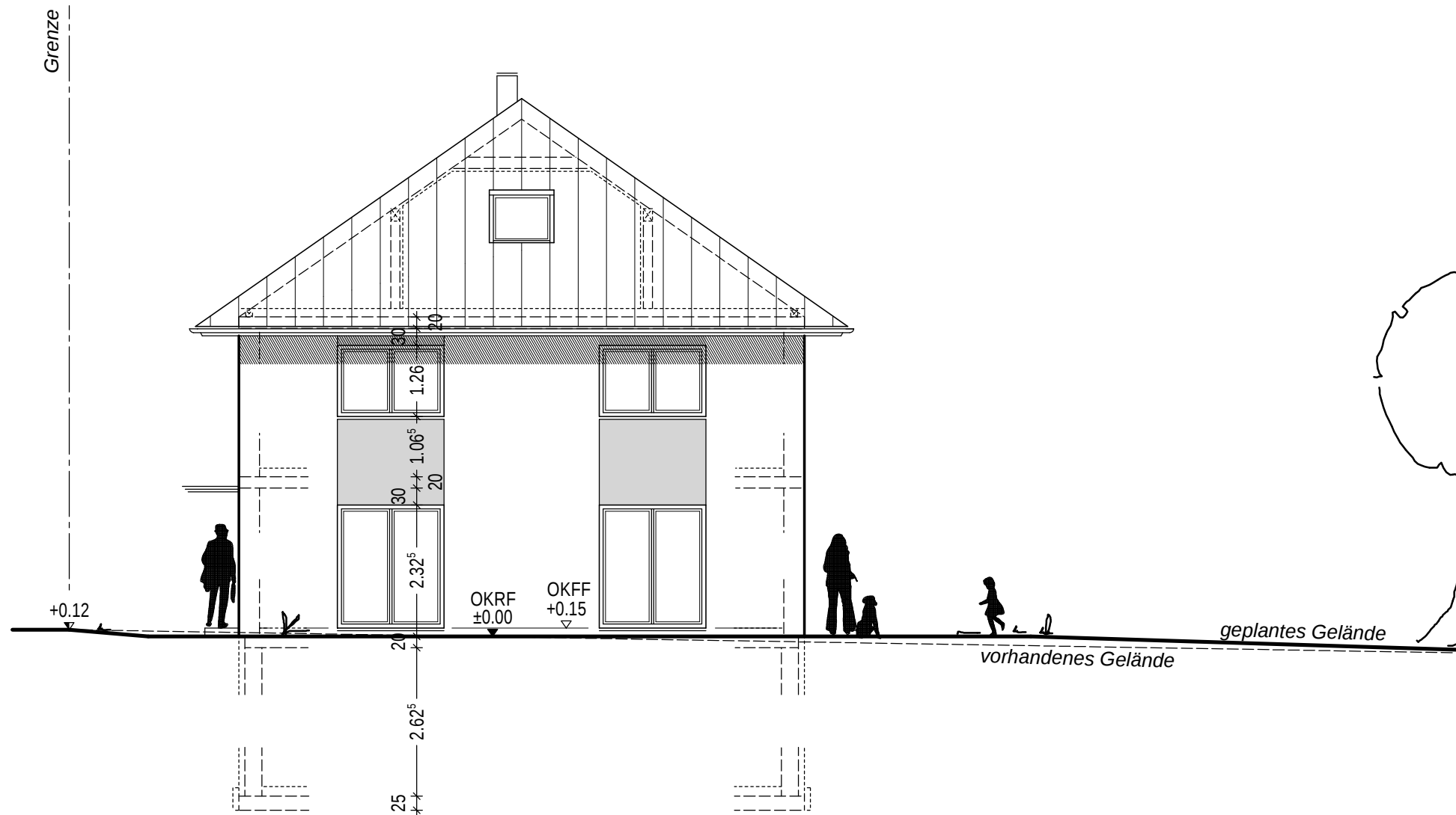
Südansicht
