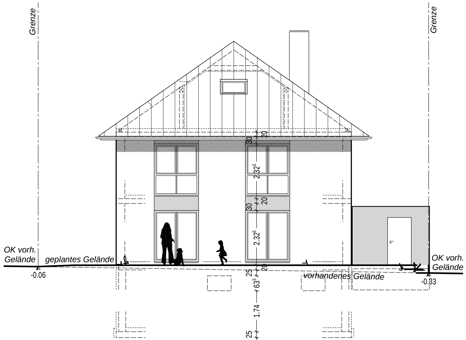
Ostansicht
