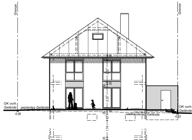
Ostansicht
