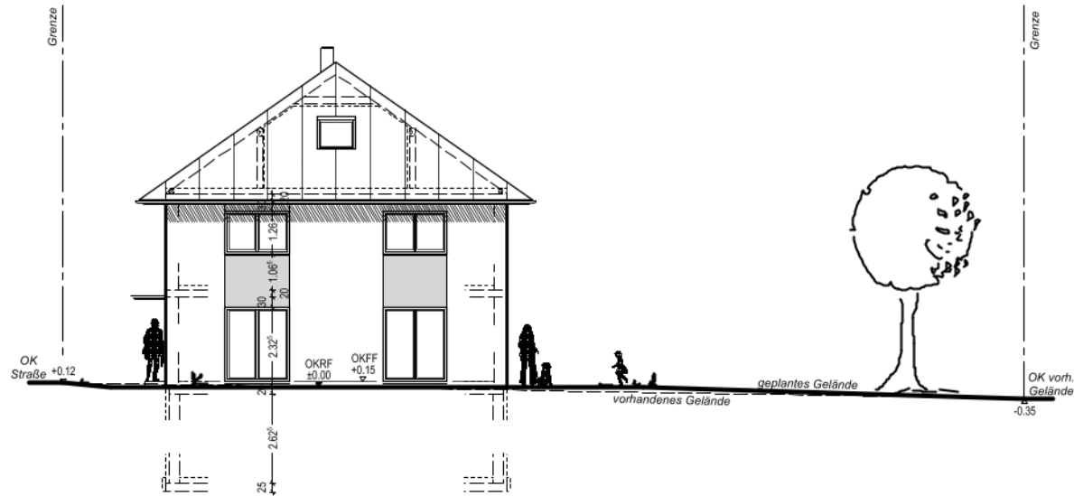
Südansicht
