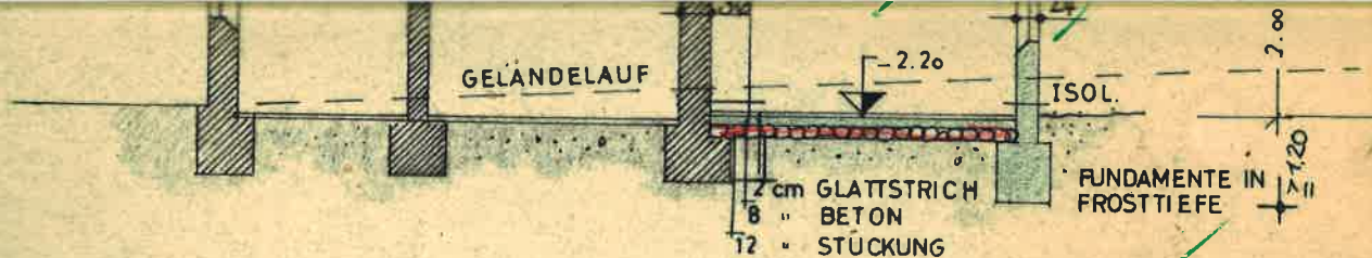
SCHNITT AB
