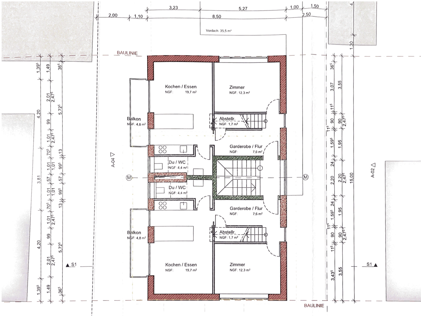
Grundriss OG
