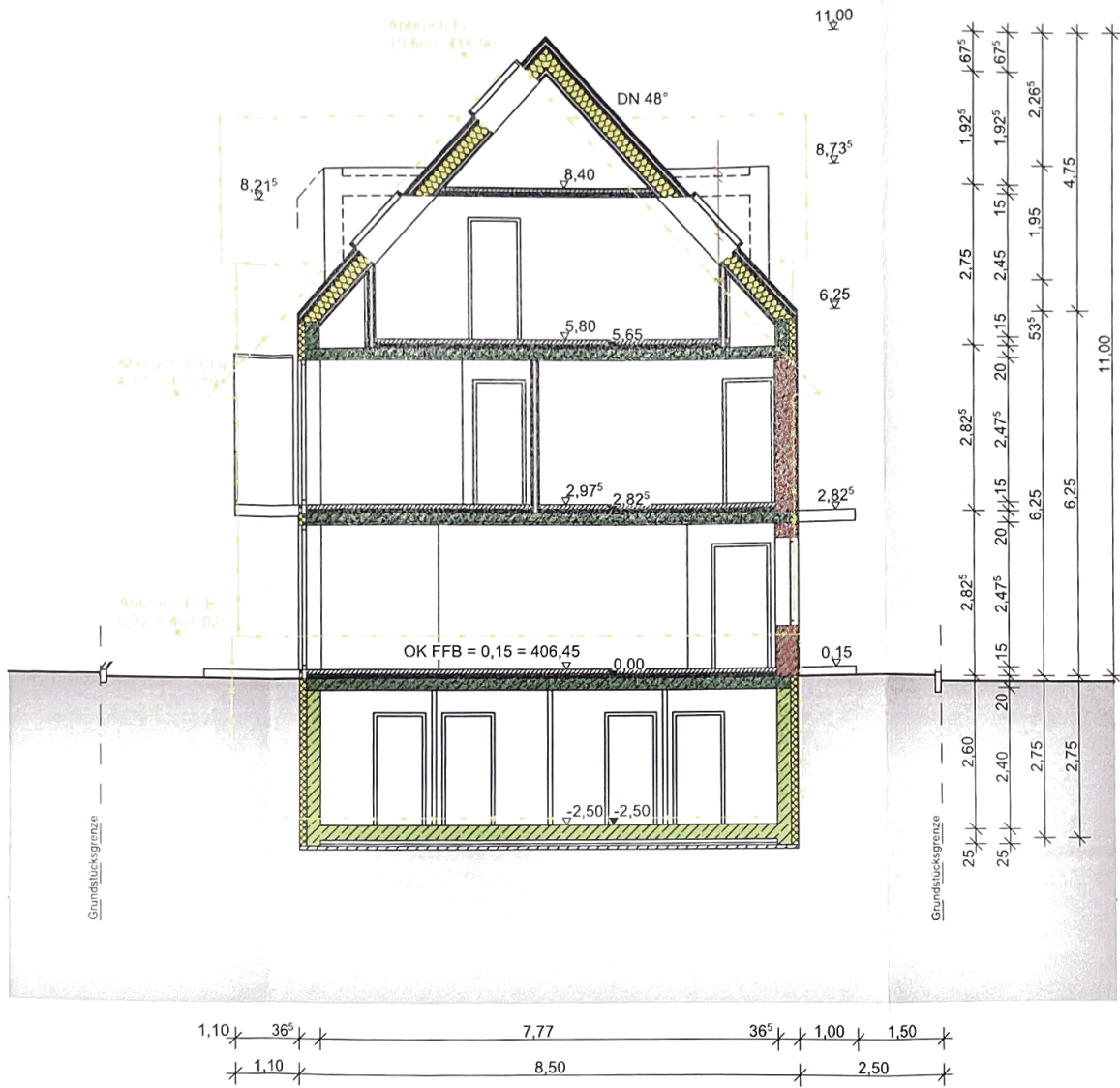
Gebäudeschnitt
