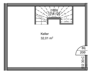
Kellergeschoß
