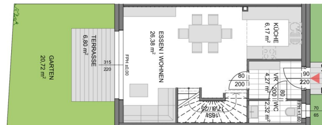
Erdgeschoss
