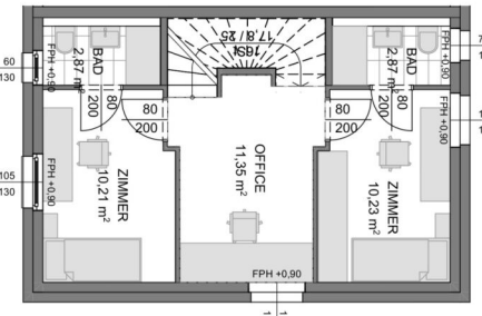
Obergeschoß
