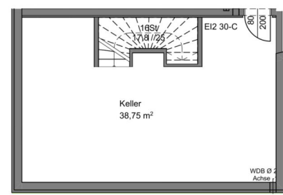
Kellergeschoss
