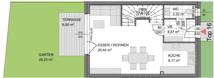
Erdgeschoss
