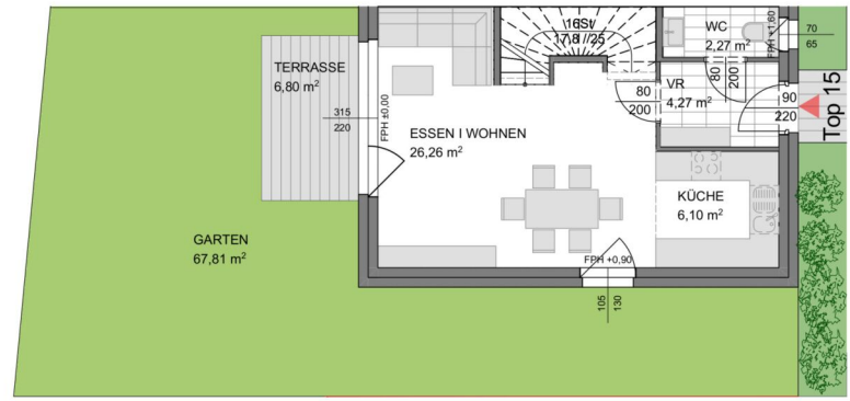
Erdgeschoss
