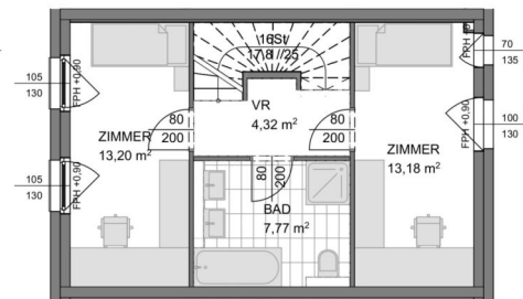
Obergeschoss
