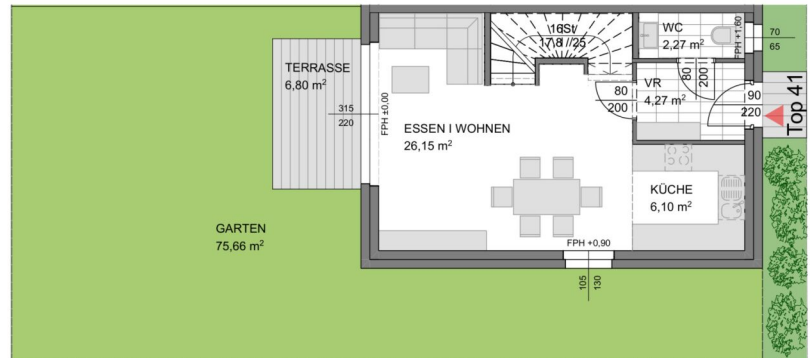
Erdgeschoss
