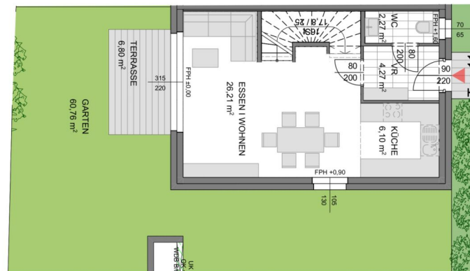
Erdgeschoss
