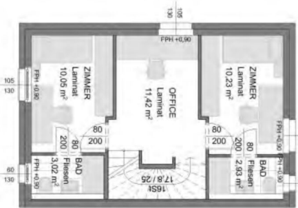
Obergeschoß
