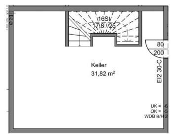
Kellergeschoß
