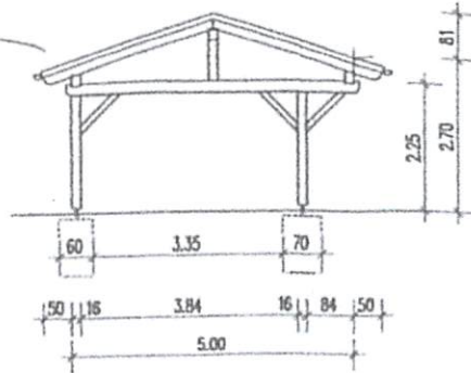
SCHNITT Überdachung 2
