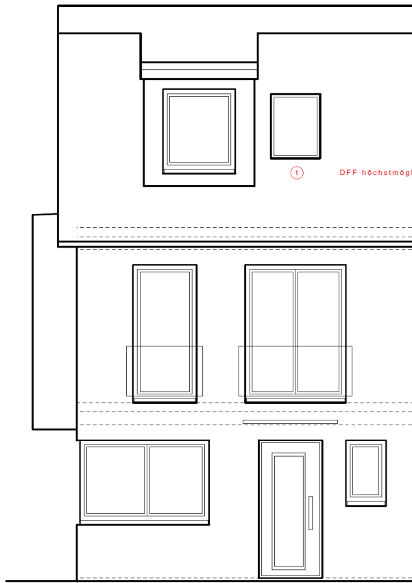
DHH - Nordansicht
