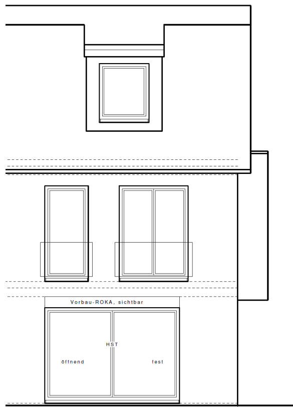
DDH - Südansicht
