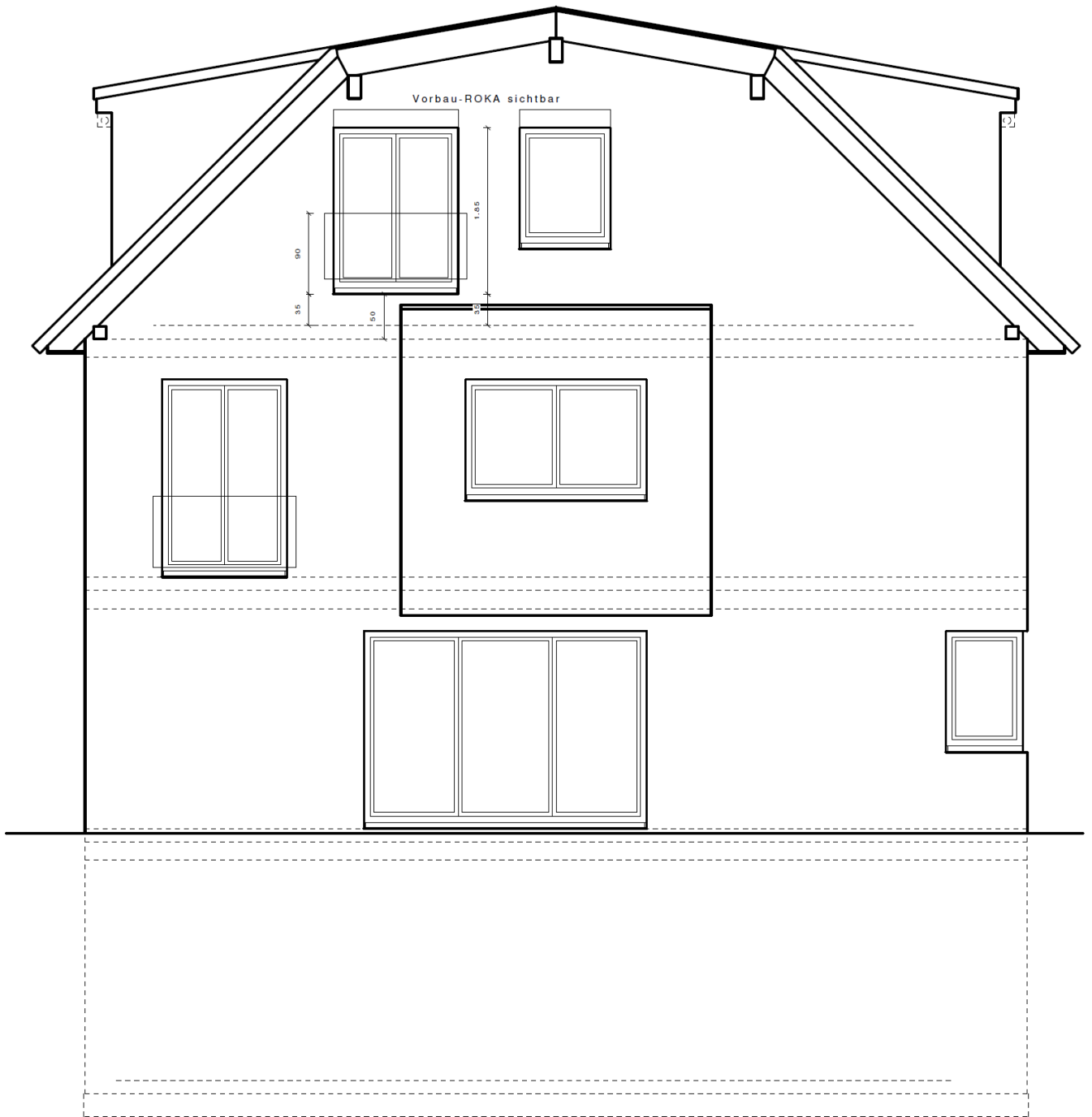
Ostansicht Haus 4
