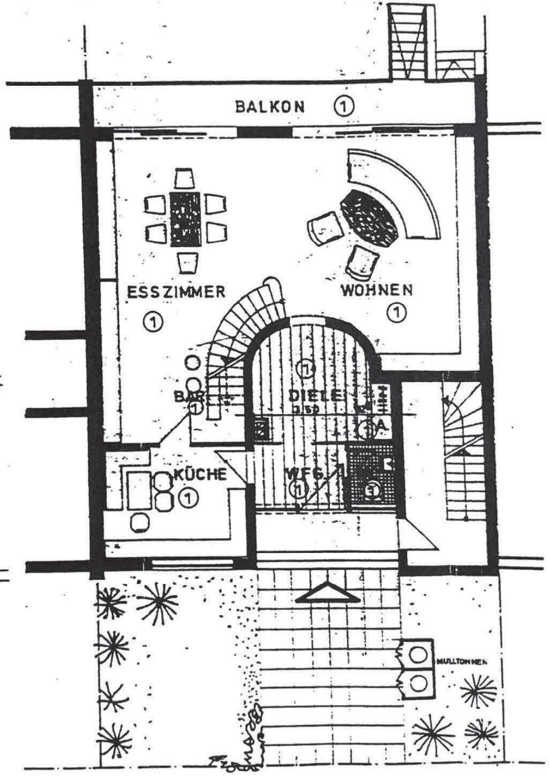
ERDGESCHOSS
