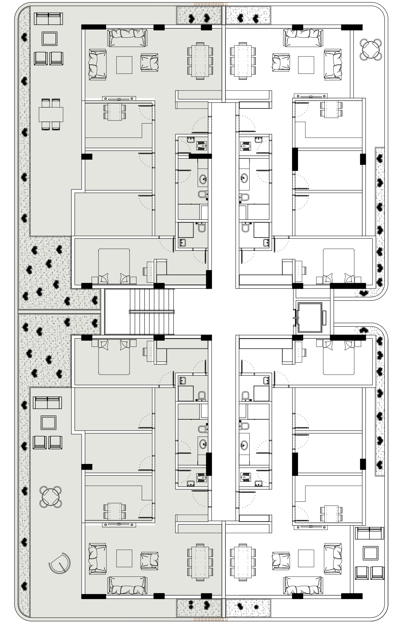
KAT PLANI
