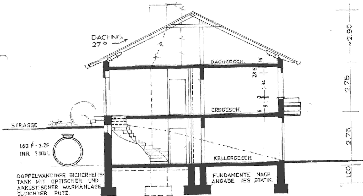
SCHNITT
