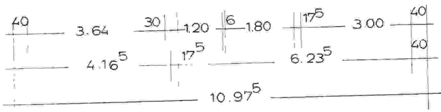
KELLERGEOSCHOSS
