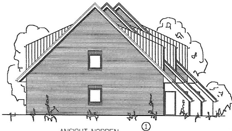
ANSICHT NORDEN
