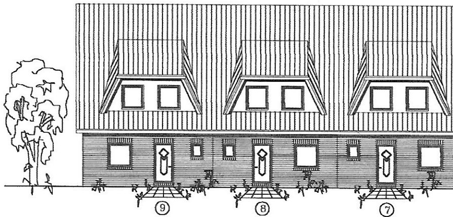
ANSICHT OSTEN
