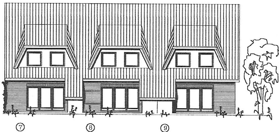
ANSICHT WESTEN
