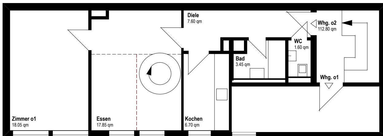
- Maisonettewohnung | 1. Obergeschoss | Ebene 1 -
