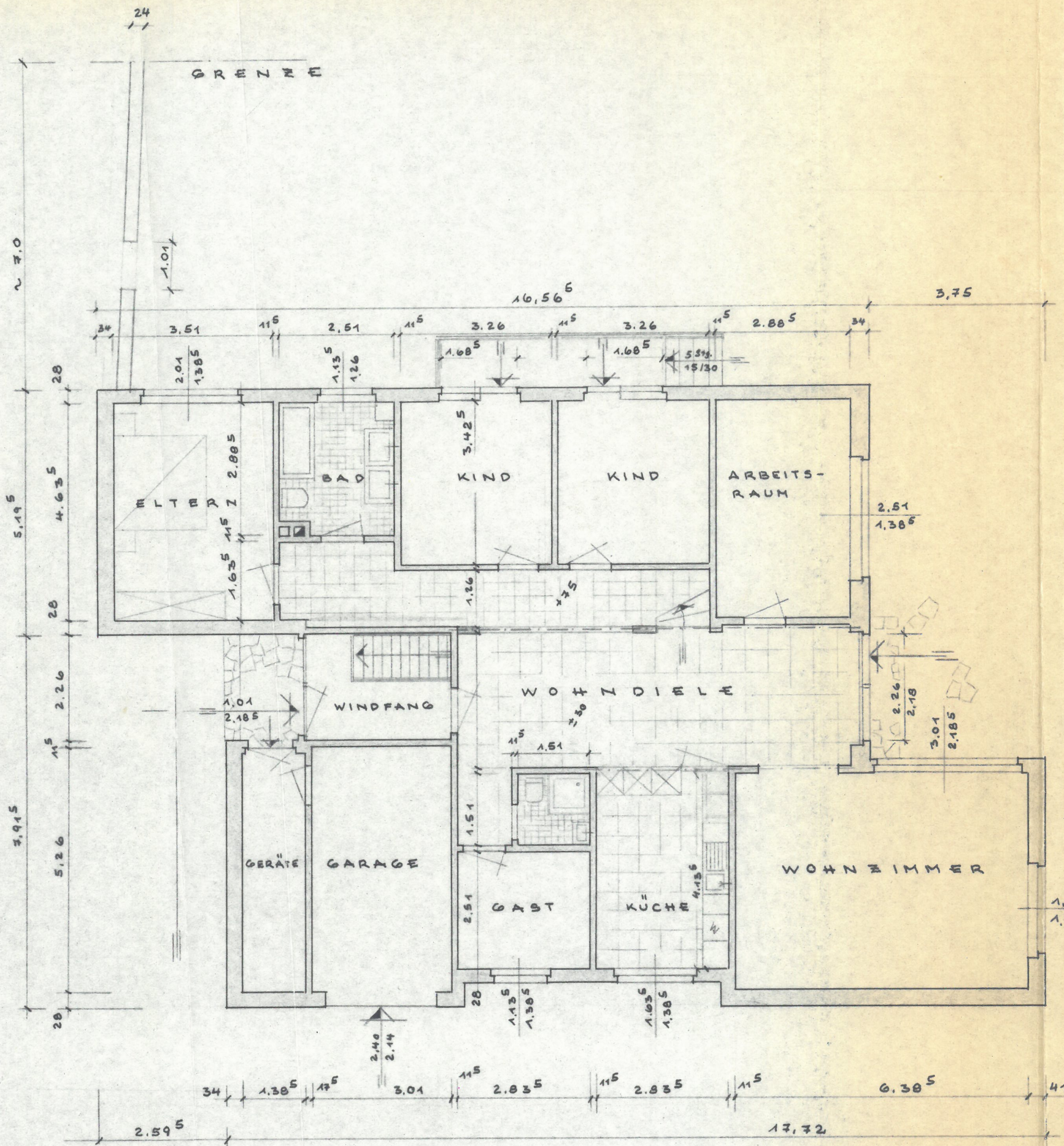
ERDGESCHOSS - GRUNDRISS
