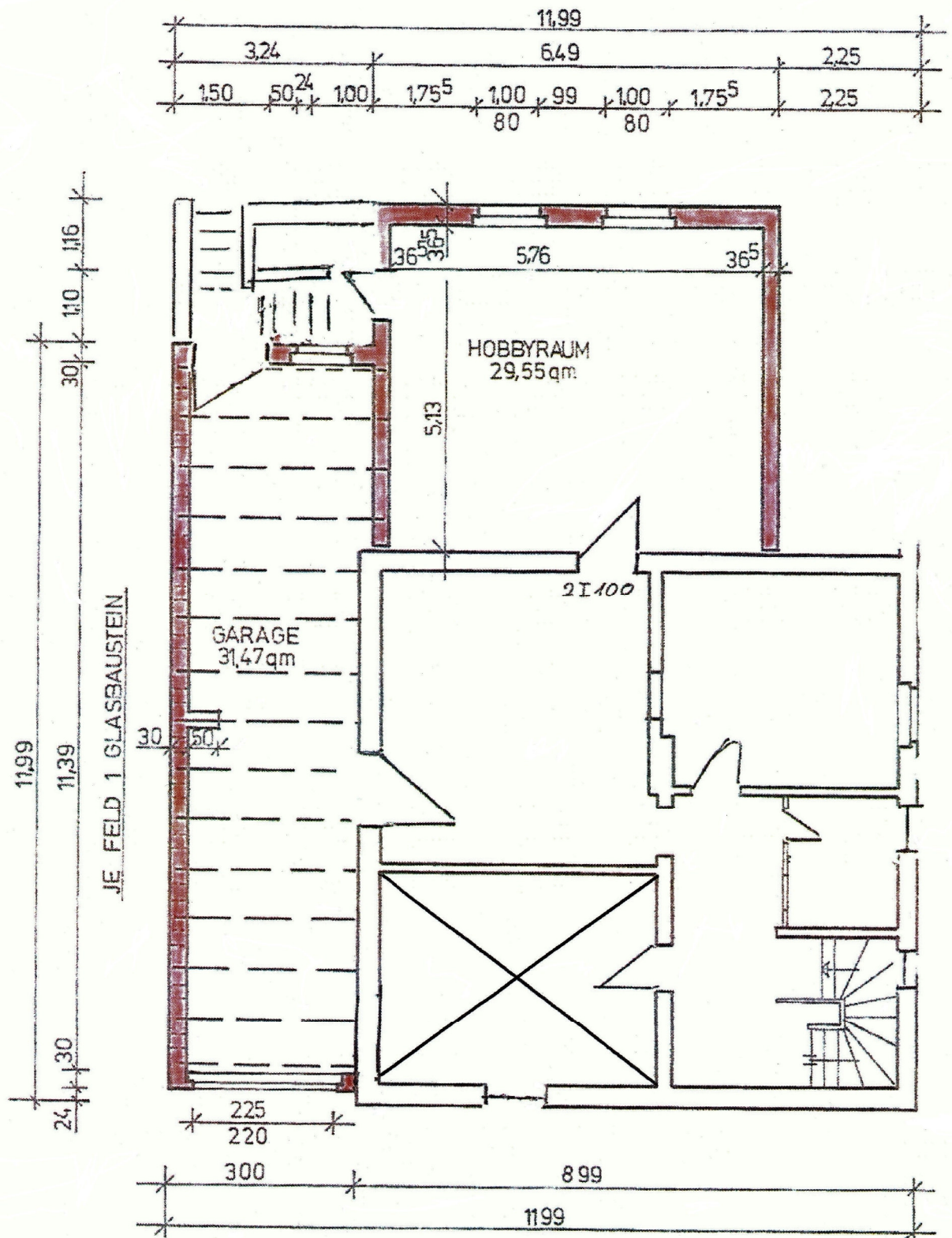
GRUNDRISS KELLERGEOSCHOS
